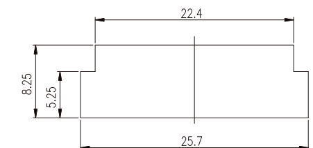
安装基准
